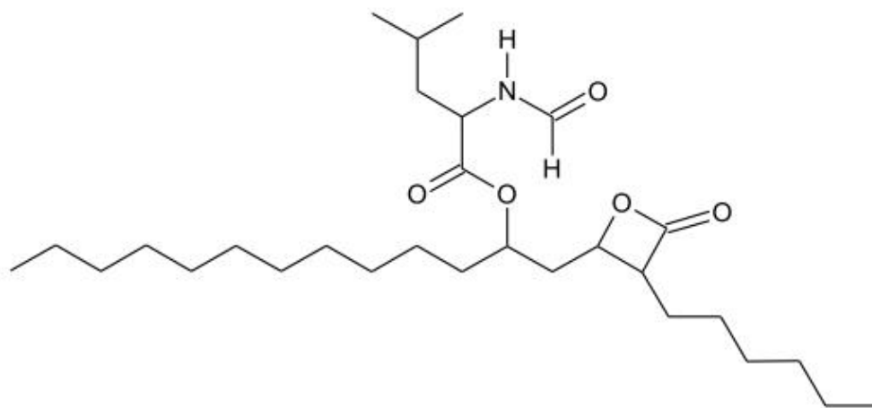
Orlistats kemiske struktur.
