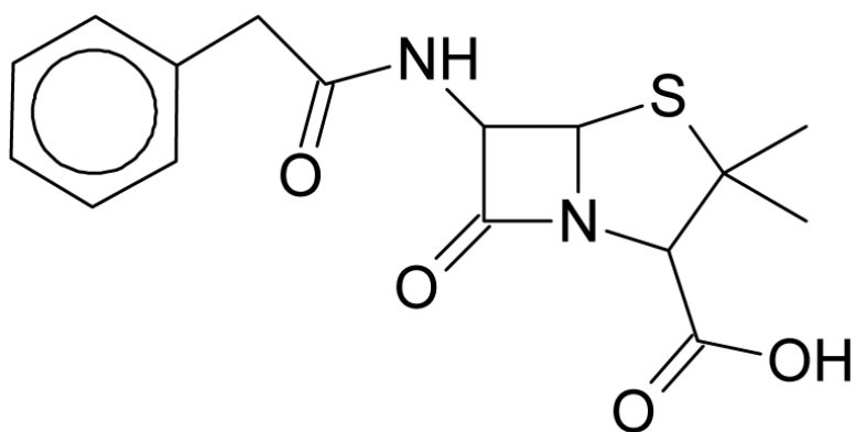
Kemisk struktur af penicillin G
